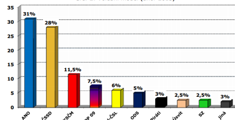
Graf 2: Volební model (únor 2015)
